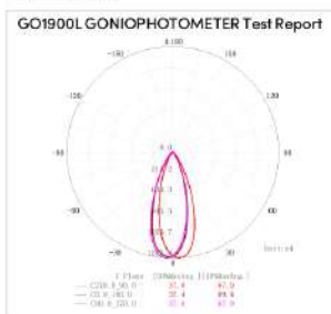
36°-3000K
